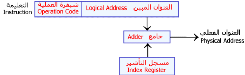
الشكل 1-20 طريقة الحصول على العنوان الفعلي في العنوان المؤشرة
